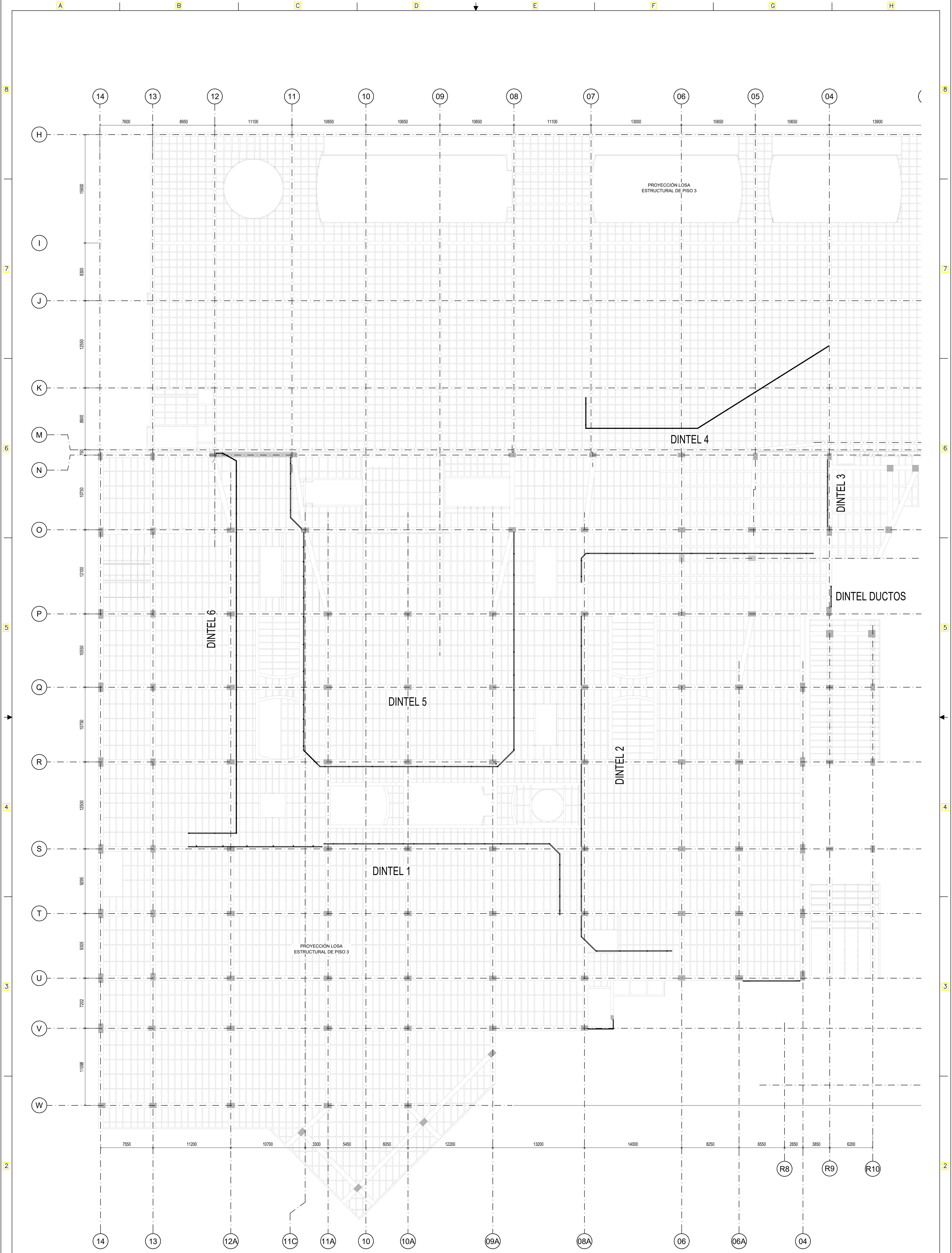
PLANTA GENERAL DINTELES PISO 2 ESCALA 2:250
