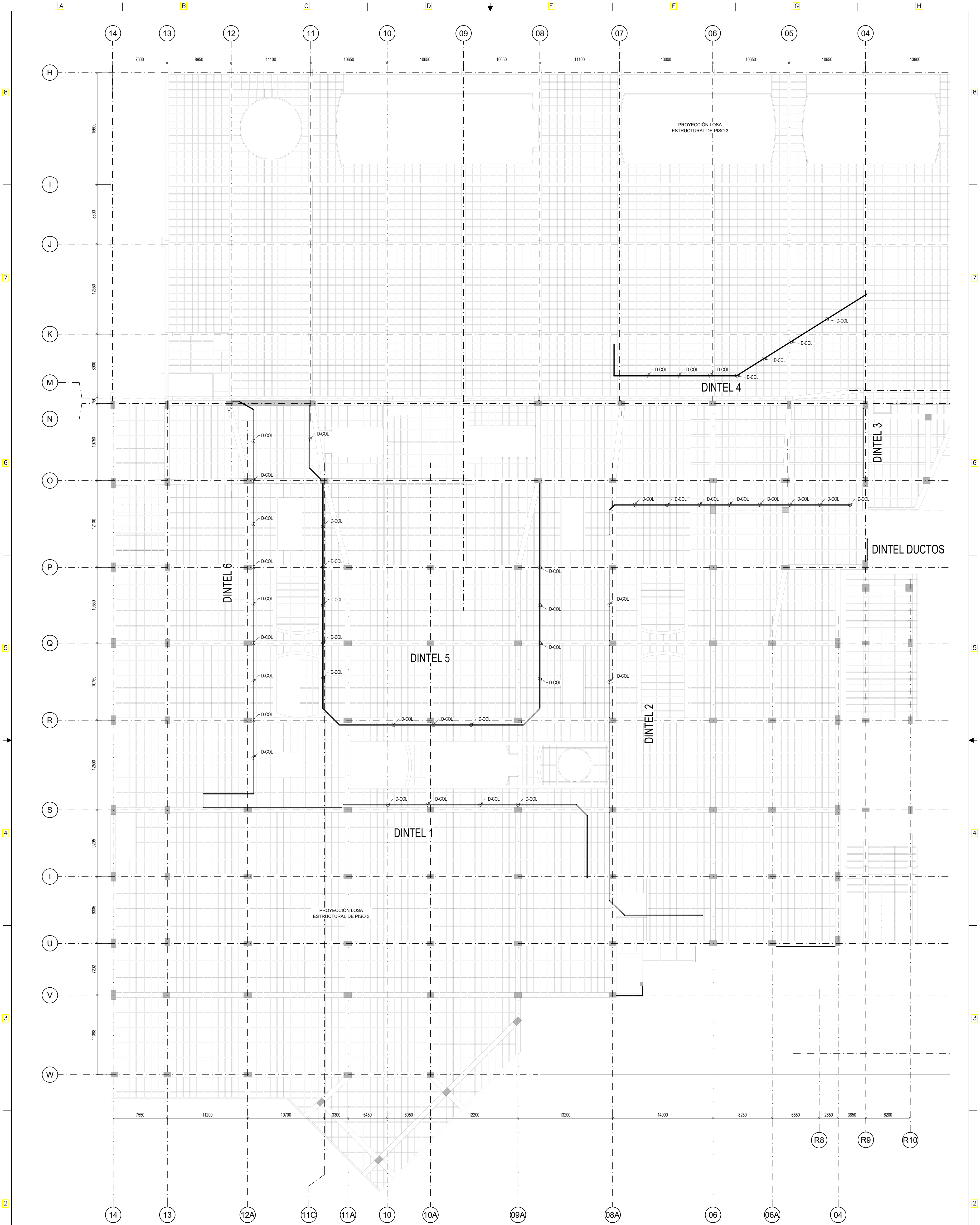
PLANTA GENERAL DINTELES PISO 2 ESCALA 2:250
